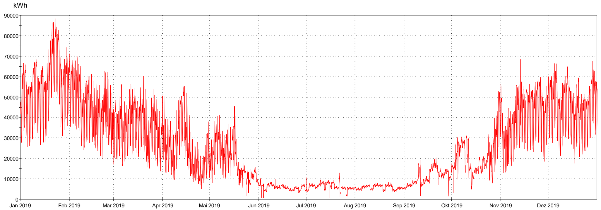
Jahreshöchstlast 88.353 kW - Lastverlauf als stündliche Leistungsmessung (Maximum am 23.01.2019 08:00 Uhr)
