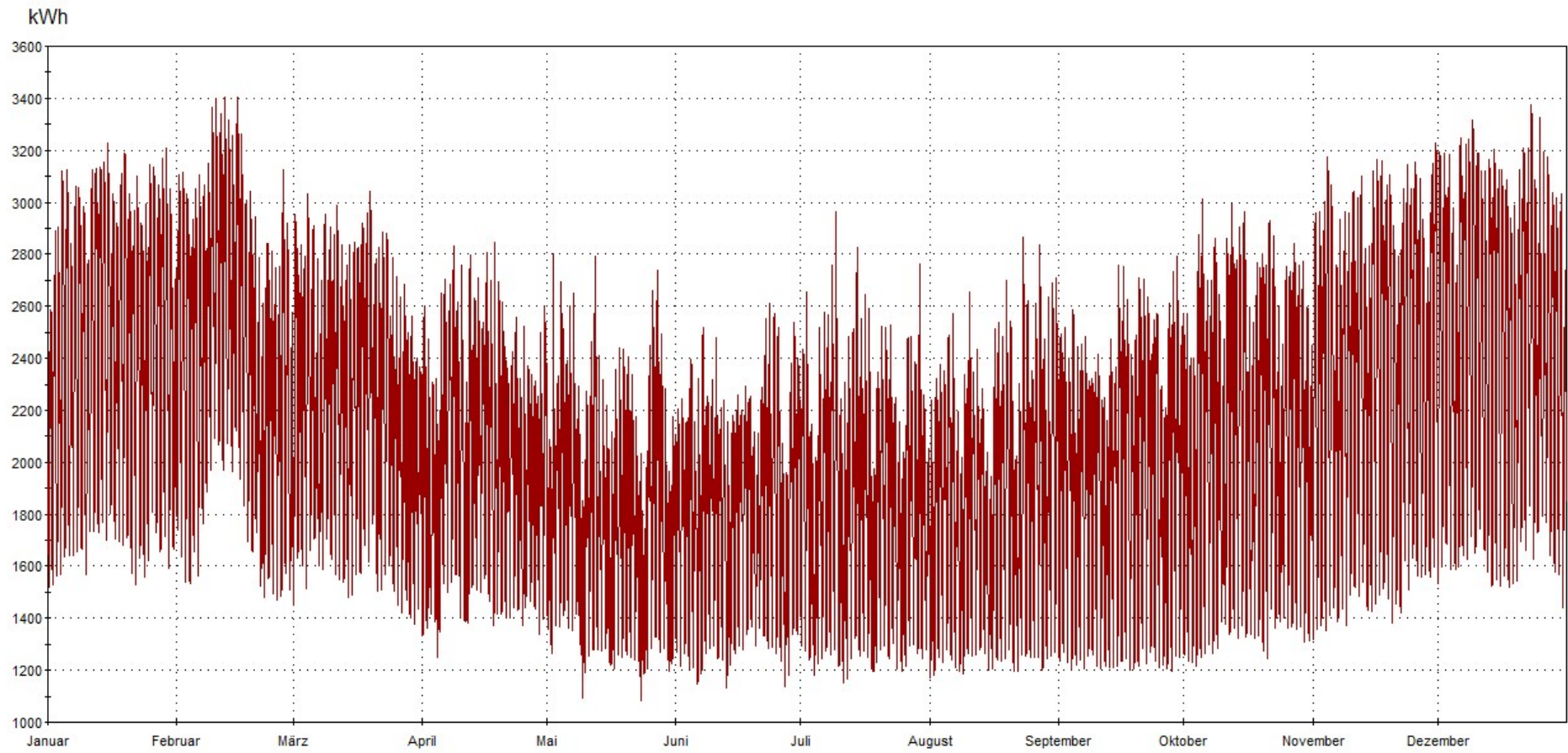
Jahreshöchstlast 13.621 kW, 12.02.2021 11:30 Uhr - Lastverlauf als viertelstündliche Leistungsmessung
