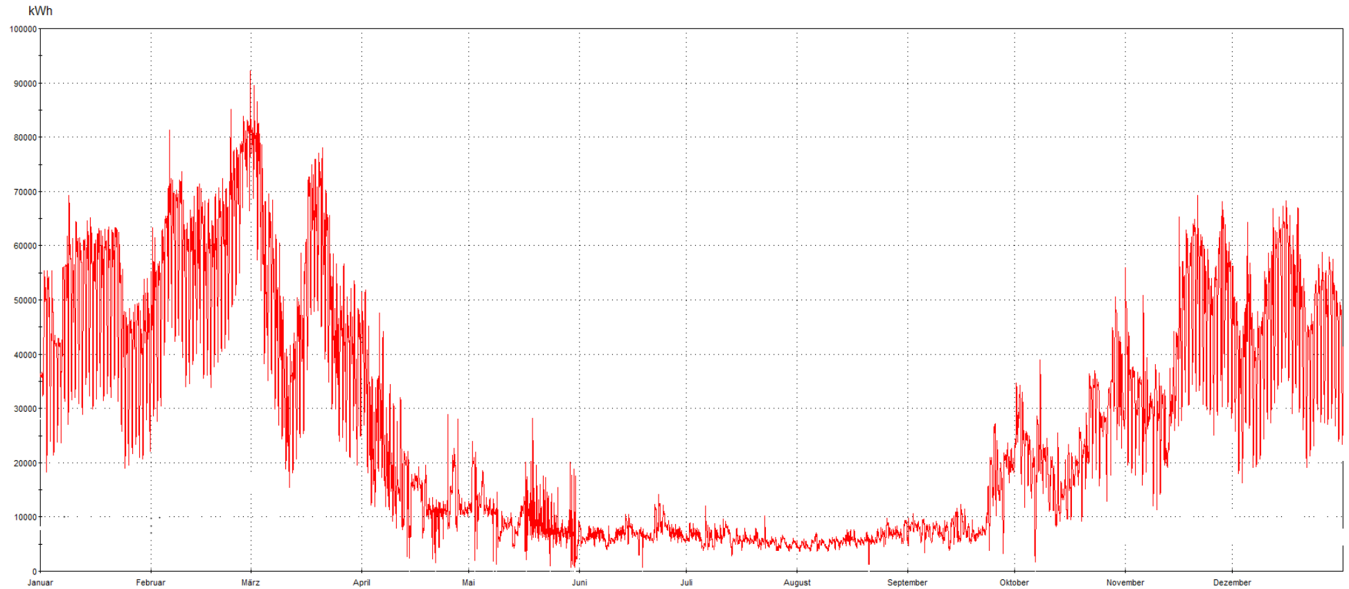
Jahreshöchstlast 92.145 kW – Lastverlauf als stündliche Leistungsmessung (Maximum am 01.03.2018 03:00 Uhr)
